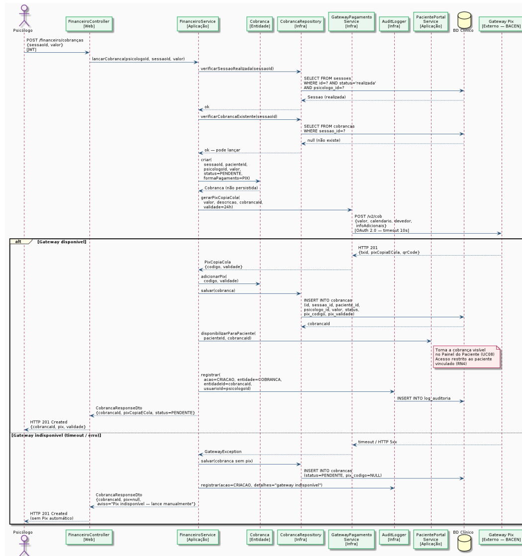
Figura: C4 — Sequência: FinanceiroService.lancarCobranca()
